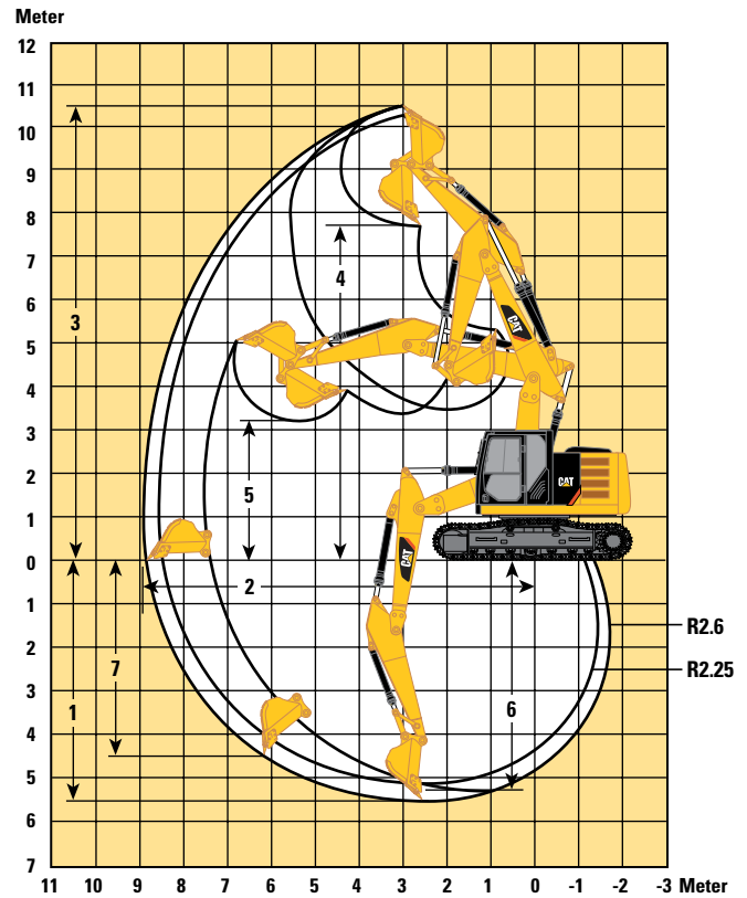
Standardausleger 5,1 m
